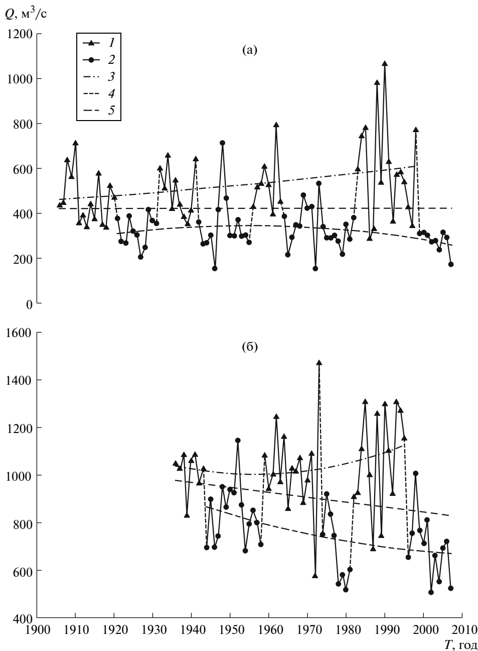
Рис. 2. Тенденции многолетних изменений стока р. Шилка у г. Сретенск (а) и р. Селенга у разреза Мостовой (б) в многогодные и маловодные фазы циклов. 1 – многоводные фазы; 2 – маловодные фазы; 3 – полиномиальный тренд многогодных фаз; 4 – полиномиальный тренд маловодных фаз; 5 – линейный тренд общего ряда.
